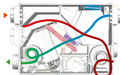
Flusso free cooling
