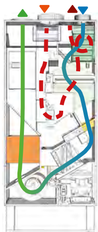
Flusso ricambio dell'aria
