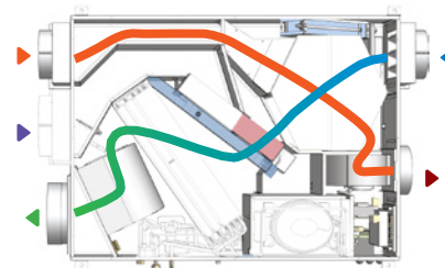
Flusso free cooling
