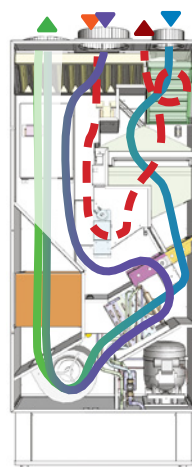
Flusso ricircolo, ricambio e trattamento aria
